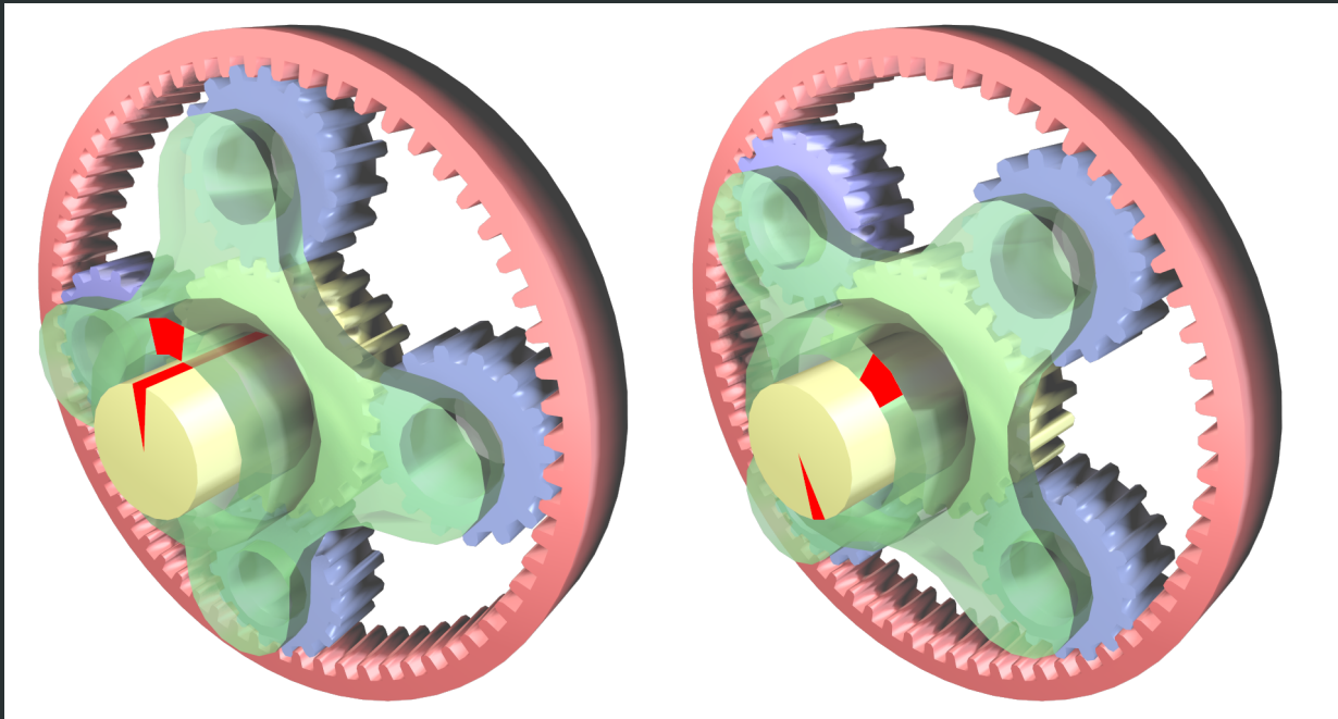
Abbildung 6.2.: Planetengetriebe mit Sonnenrad (gelb), Planetenrädern (blau), Planetenradträger (grün) sowie Hohlrads (rot). Das rechte Bild zeigt die relative Verschiebung von Sonnenrad und Planetenradträger, nachdem letzterer um 45^\circ rotiert wurde. Quelle: Wikipedia
