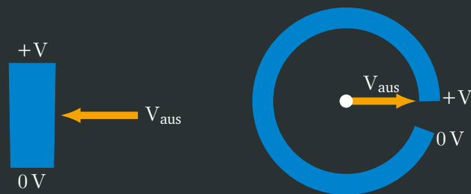
Abbildung 7.1.: Lineares (links) und rotatorisches (rechts) Potentiometer mit Widerstandselement (blau) und Kontakt (orange).
