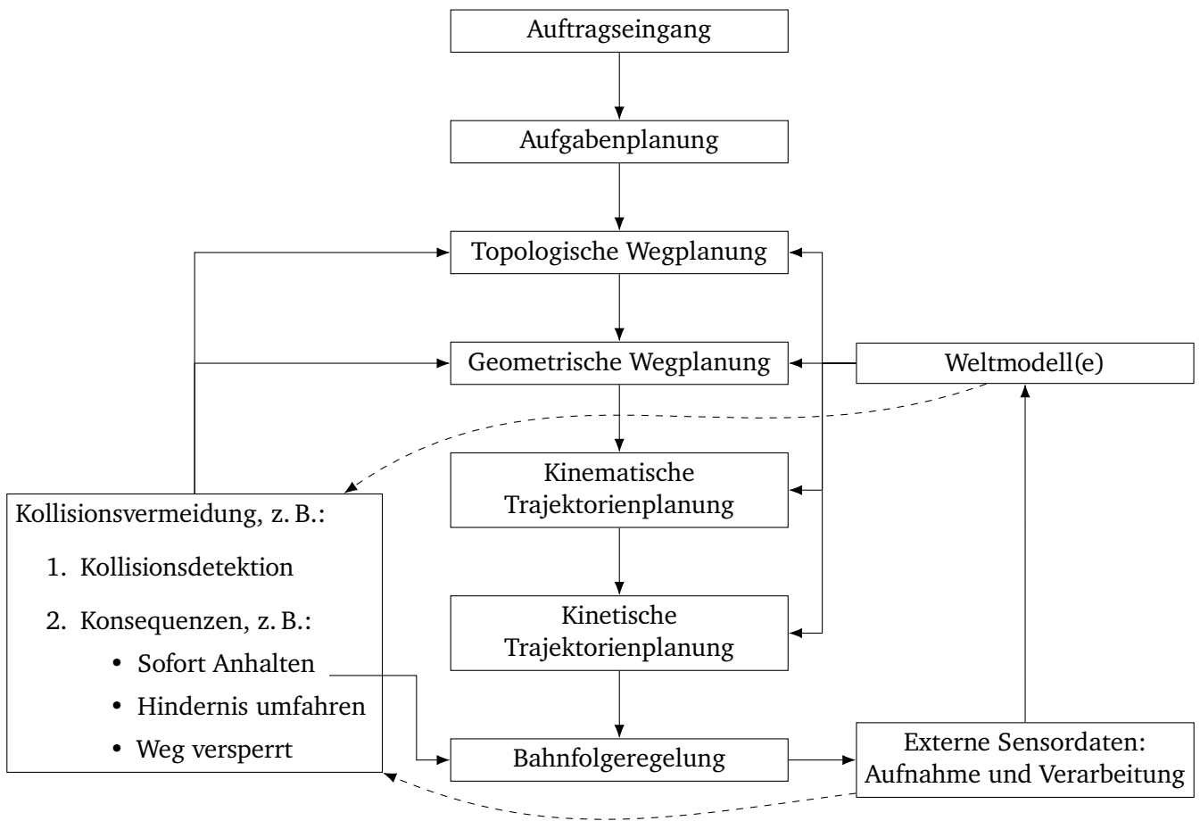
Abbildung 9.1.: Hierarchische Auftragsbearbeitung und Planung.
