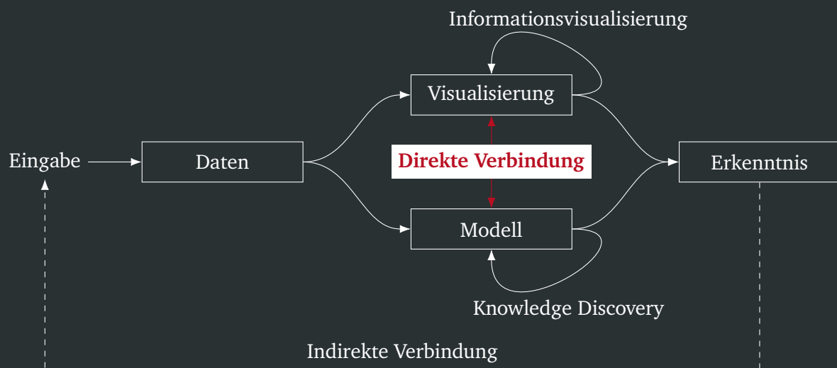
Abbildung 4.4: Das Visual Analytics Prozessmodell
