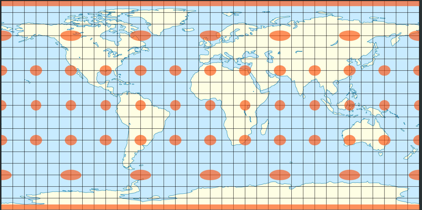
Abbildung 3.17: Verzerrung durch die Plattkarten-Projektion
