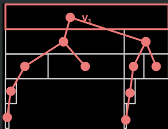
(a) Icicle-Plot
