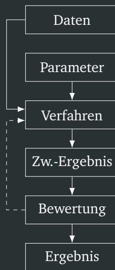
Abbildung 4.5: Darstellung der grundlegenden Schritte von automatischen Verfahren. Das Zwischenergebnis hat dabei häufig, aber nicht immer, die gleiche Form wie das Ergebnis, wird allerdings iterativ verändert. Hat es die gleiche Form, so können die selben Visualisierungstechniken für das Zwischenergebnis wie für das Ergebnis angewendet werden.
