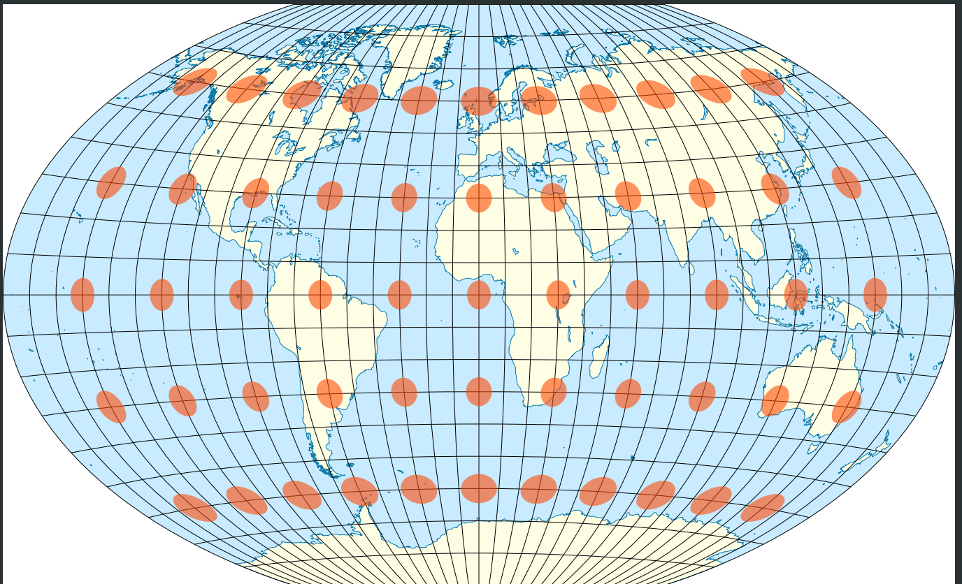
Abbildung 3.19: Verzerrung durch die Winkel-Tripel-Projektion
