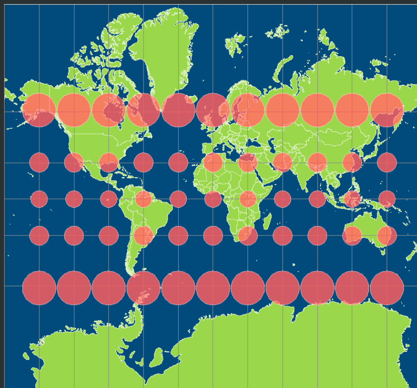
Abbildung 3.18: Verzerrung durch die Mercator-Projektion
