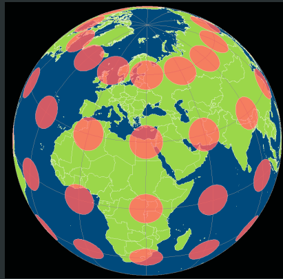
Abbildung 3.16: Tissotsche Indikatrix auf dem Globus
