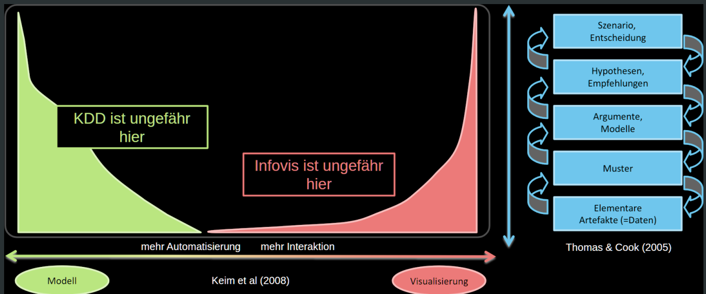
Abbildung 4.3: Die zwei Achsen der Visual Analytics Quelle: Vorlesungsfolien
