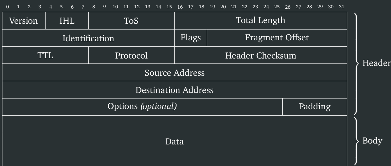
Abbildung 5.1: IPv4 Paketformat
