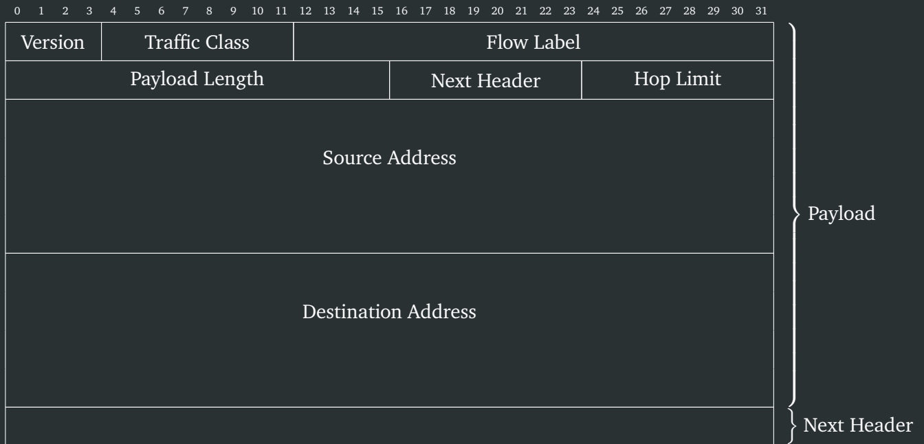
Abbildung 5.3: IPv6 Paketformat
