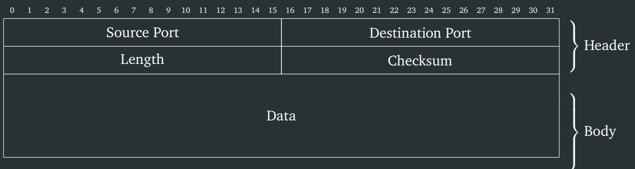
Abbildung 6.7: UDP Paketformat
