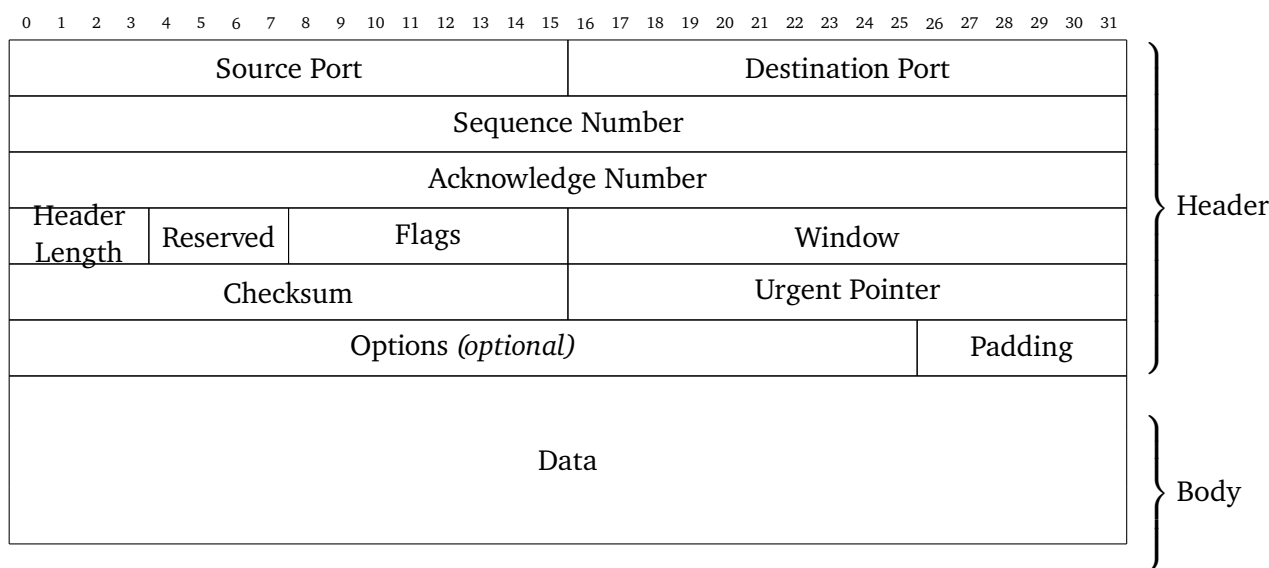
Abbildung 6.8: TCP Paketformat
