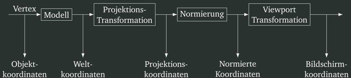
Abbildung 8.1.: Änderung der Koordinaten innerhalb der Grafikpipeline.
