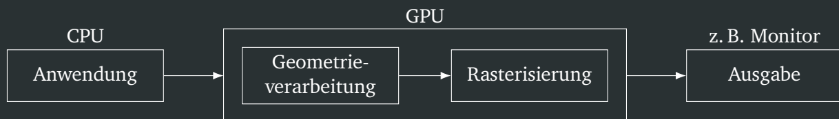
Abbildung 7.3.: Typische Grafikpipeline
